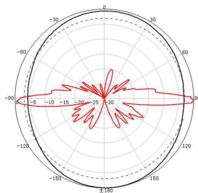
H-Pol @ 2450MHz
