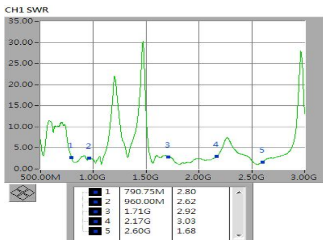
VSWR
